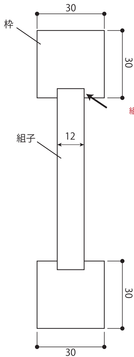
枠 30mm×30mm
